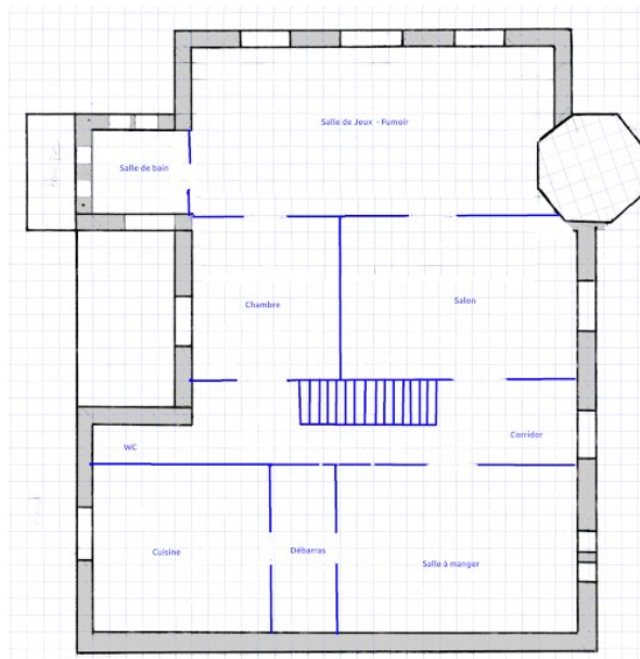
Figure 55: Regina Caeli : plan du rez-de-chaussée
