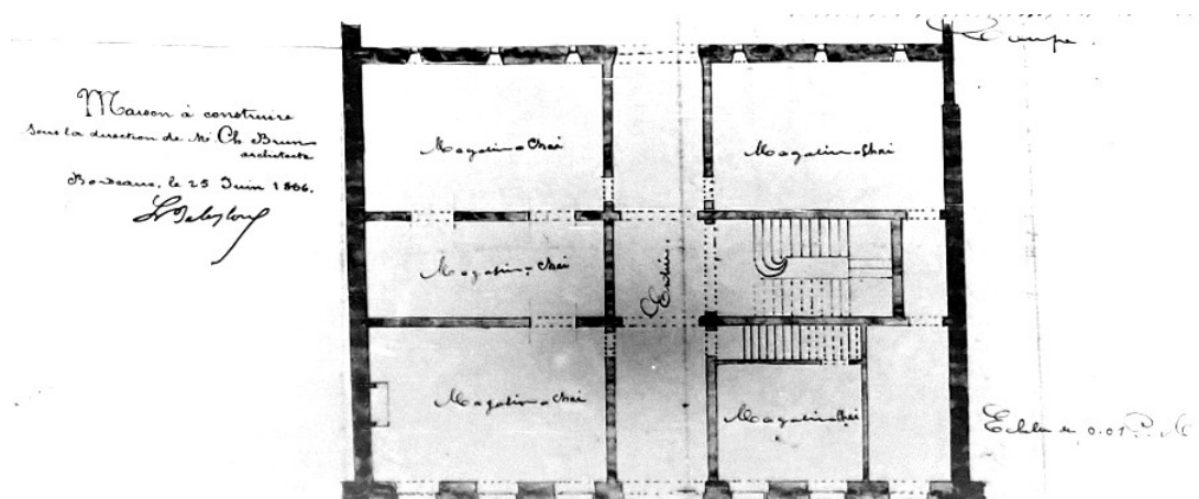
Figure 39: Plan du sous-sol de l'Hôtel rue Castéja : source ABM
